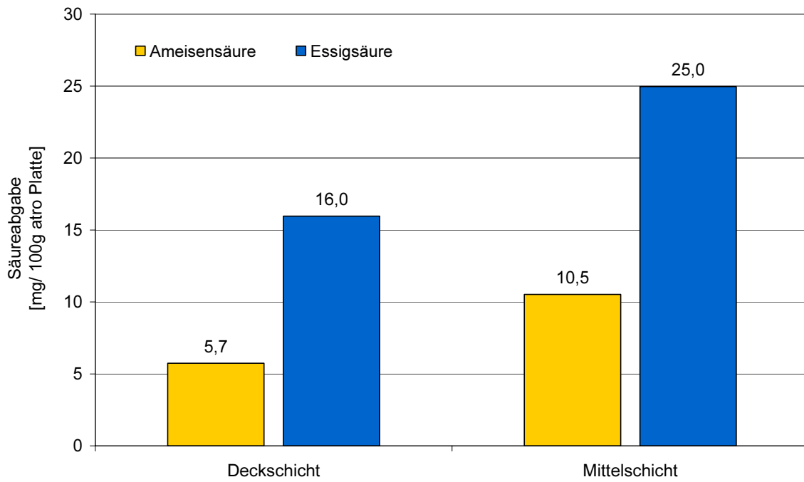
Abbildung 1: Abgabe von Ameisen- und Essigsäure aus Deck- und Mittelschichten von aus CTMP hergestellten MDF
