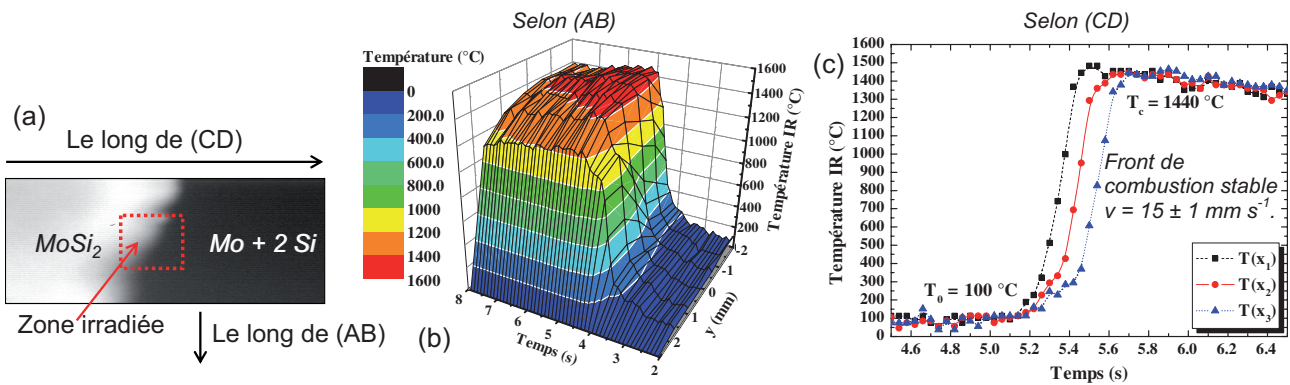
Fig. 4. Analyse thermique de la réaction de Mo + 2 Si \rightarrow MoSi_2 : (a) image macroscopique du front de propagation au cours de la réaction SHS initiée par un courant électrique, (b) analyse thermique le long de l'axe (AB) perpendiculaire à au front de combustion au milieu de l'échantillon, (c) trois thermogrammes enregistrés le long de l'axe (CD) du front de combustion aux positions x_1, x_2 et x_3 .
