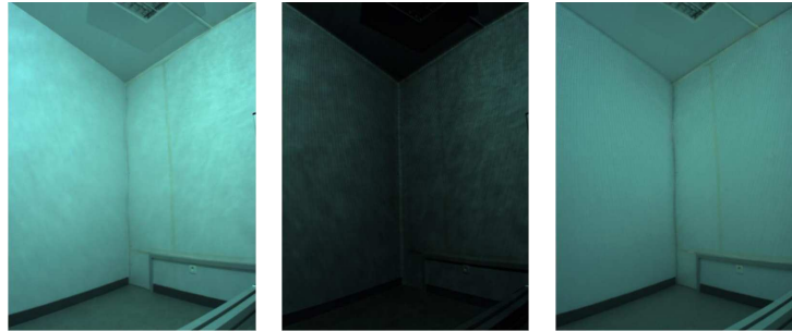
Figure 2: Gauche : scène réelle visible lors de la projection immersive par l'avant d'une image blanche. Milieu : éclairage réfléchi directement, du projecteur vers la caméra, correspondant. Droite : éclairage réfléchi indirectement, après réflexions multiples, correspondant.
