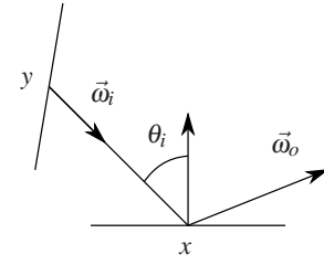
Figure 3: Notations pour l'équation de luminance.
