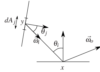
Figure 4: Notations pour l'équation de radiativité.
