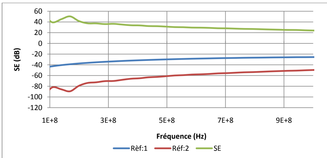
Fig.9. L'efficacité du blindage électromagnétique en transmission de film d'argent AgHT-4.
