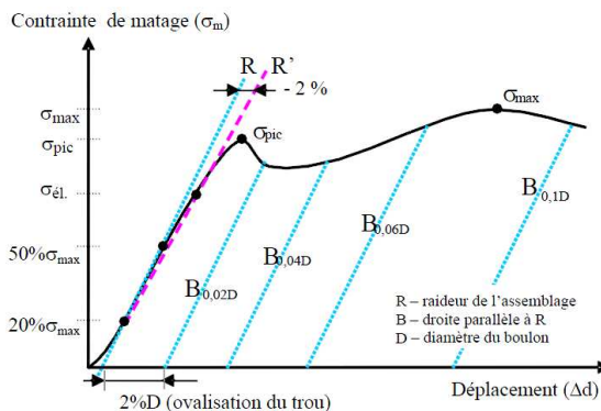
Fig. 10 Courbe type d'un essai de matage [11]
