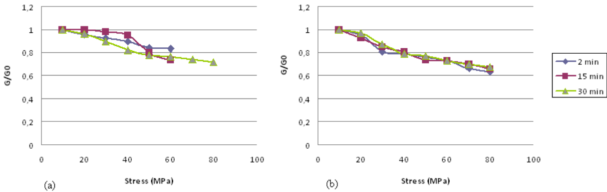
Fig. 6. Influence du temps de relaxation sur l'évolution du module de cisaillement : (a) Carbestamp® PA 12 (b) Carbestamp® PA 6
