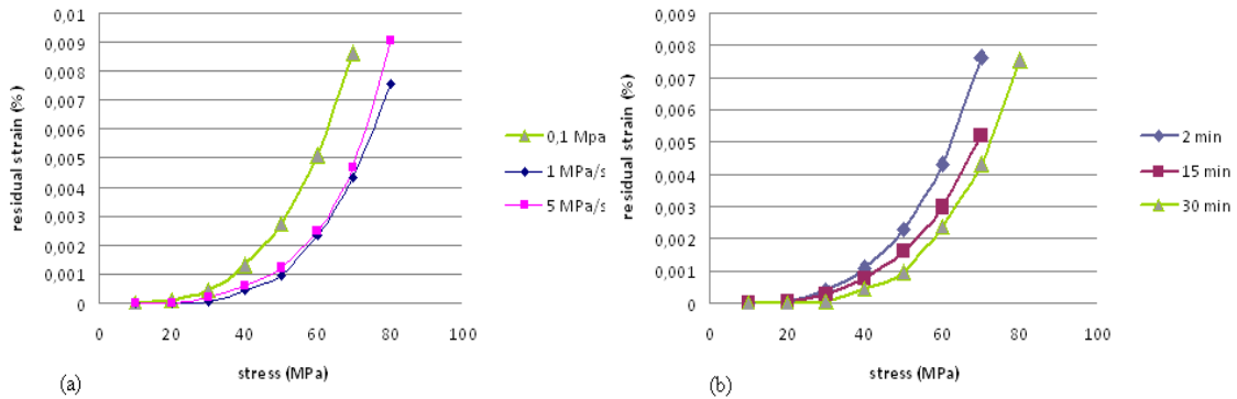
Fig.7. Influence de la vitesse de sollicitation (a) et du temps de relaxation (b) sur la deformation résiduelle lors d'essais de charge / décharges sur des stratifiés Carbestamp® PA 6 [ \pm 45 ] s
