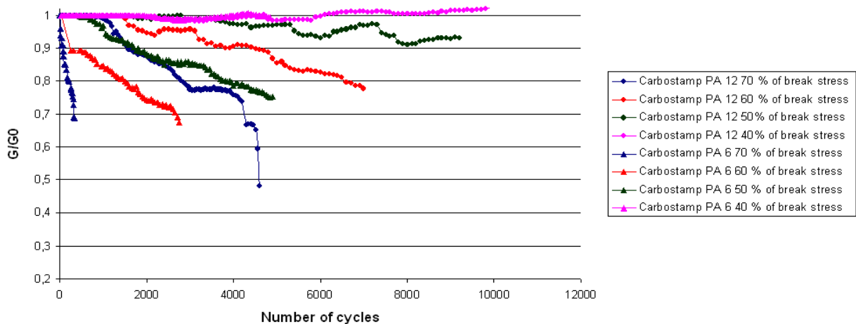
Fig. 8. Evolution du module de cisaillement avec le nombre de cycles de fatigue pour le Carbestamp® PA 6 et PA 12
