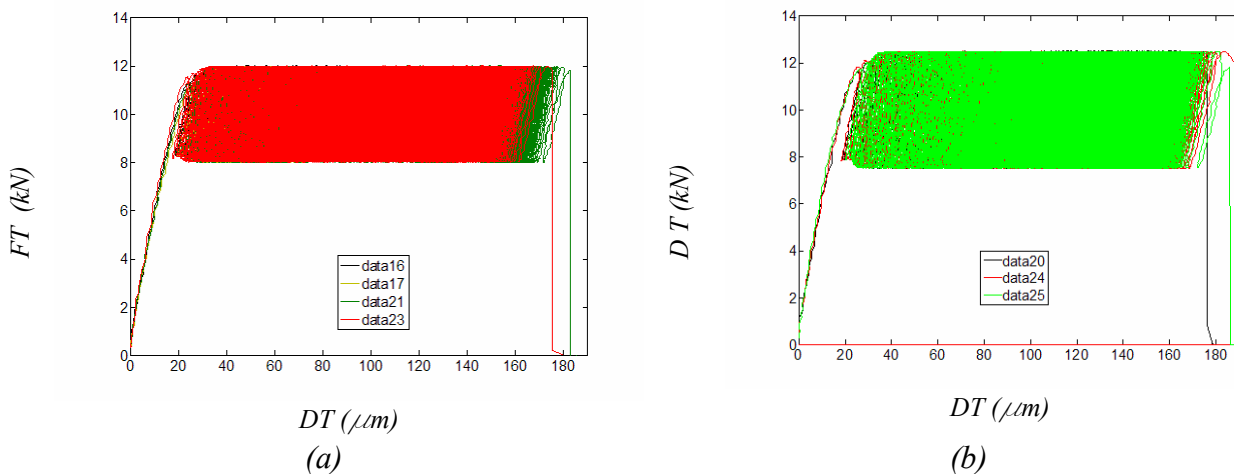
Fig. 5 : Courbes effort-déplacement sous chargement cyclique : (a) F_m=10 kN et F_a=2,0 kN (1 kN/s), (b) F_m=10 kN et F_a=2,5 kN (1 kN/s).
