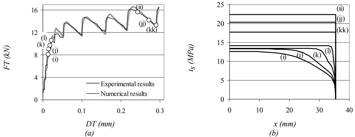
Figure 10: Réponse du modèle de Chase Goldsmith pour un essai de cisaillement de type relaxation-fluage : (a) Diagramme effort déplacement tangentiel, (b) Evolution de la distribution des contraintes dans le plan moyen du joint de colle suivant la demi-longueur de recouvrement.
