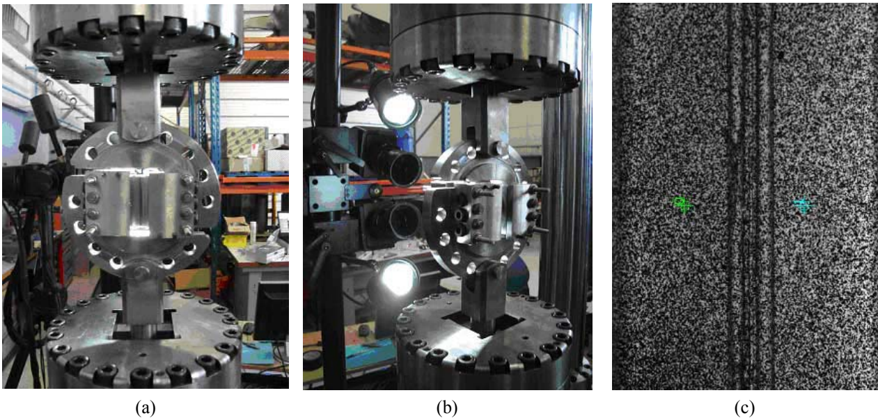
Fig. 3 : Dispositif Arcan modifié : (a) Dispositif Arcan pour un essai de cisaillement, (b) Dispositif de mesure 3D en temps réel sans contact, (c) Suivi par marqueur du déplacement des extrémités du joint de colle.
