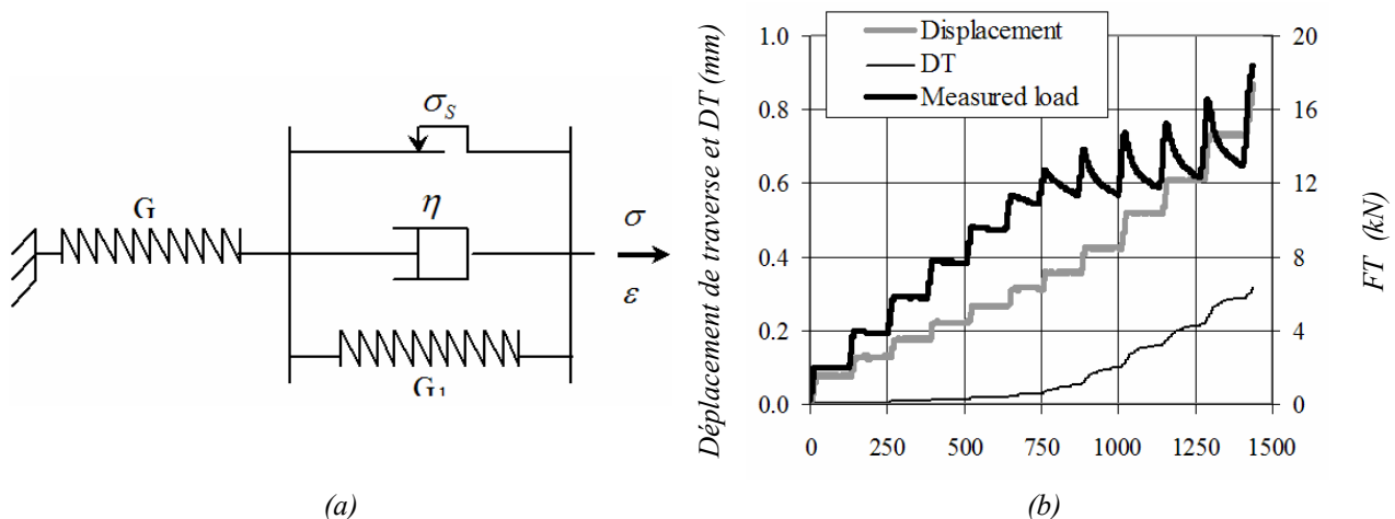
Fig. 9 : Modèle de Chase Goldsmith avec viscosité non-linéaire : (a) Formulation analogique, (b) Réponse expérimentale pour une sollicitation de relaxation-fluage (vitesse de déplacement de la traverse=0,5 mm/min).
