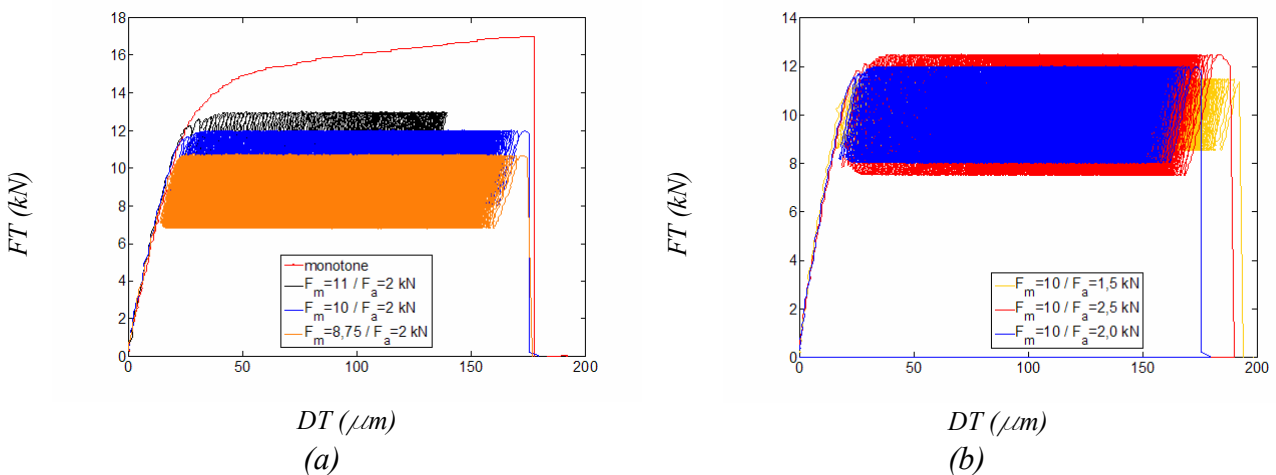
Fig. 7 : Courbes déplacement-temps sous chargement cyclique : (a) Influence de la charge moyenne, (b) Influence de la charge alternée.
