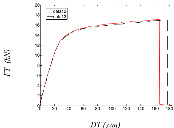
Fig. 4 : Courbes effort-déplacement sous chargement monotone (1 kN/s).
