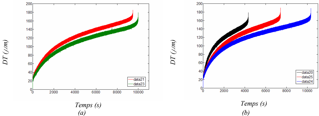
Fig. 6 : Courbes déplacement-temps sous chargement cyclique : (a) F_m=10 kN et F_a=2,0 kN (1 kN/s), (b) F_m=10 kN et F_a=2,5 kN (1 kN/s).
