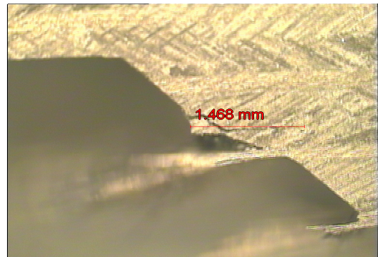
Fig. 8. Délaminage essai 19.
