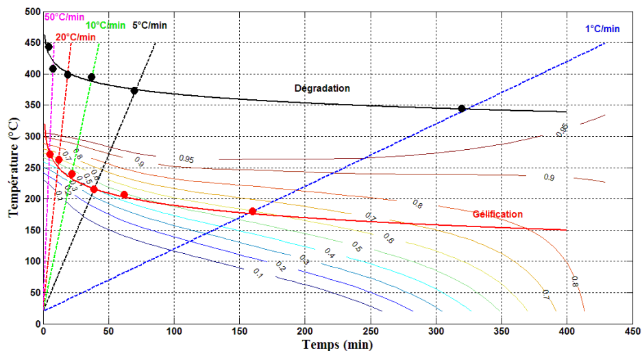
Figure 7 Diagramme TTT dynamique de la résine M21
