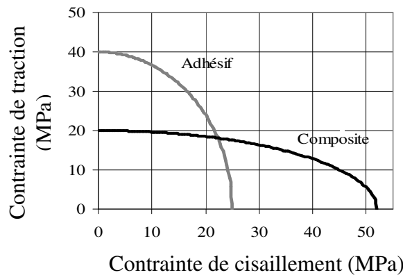
Fig. 4. Présentation schématique des limites à rupture pour la colle et le composite dans le diagramme contrainte de traction – contrainte de cisaillement.
