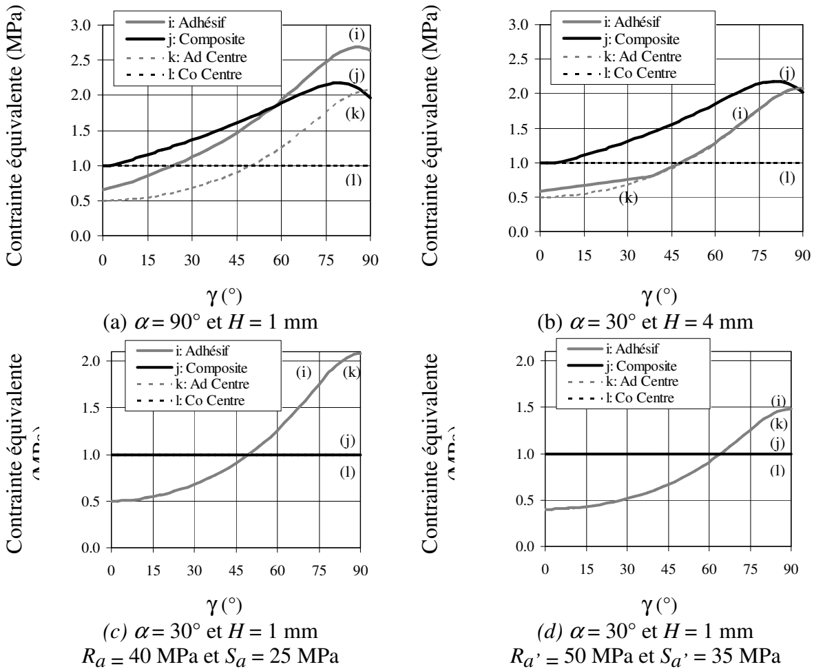
Fig. 3. Valeurs maximales des contraintes équivalentes normalisées dans l'adhésif et le composite en fonction du chargement de traction-cisaillement, \gamma \in [0^\circ, 90^\circ] ( D = 5 \text{ mm} , h = 0.2 \text{ mm} , bords nettoyés \rho = 1.5 * h ).
