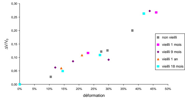
Fig.14. Suivi de l'endommagement par variation relative de volume du matériau C après différentes durées de vieillissement à 80°C.
