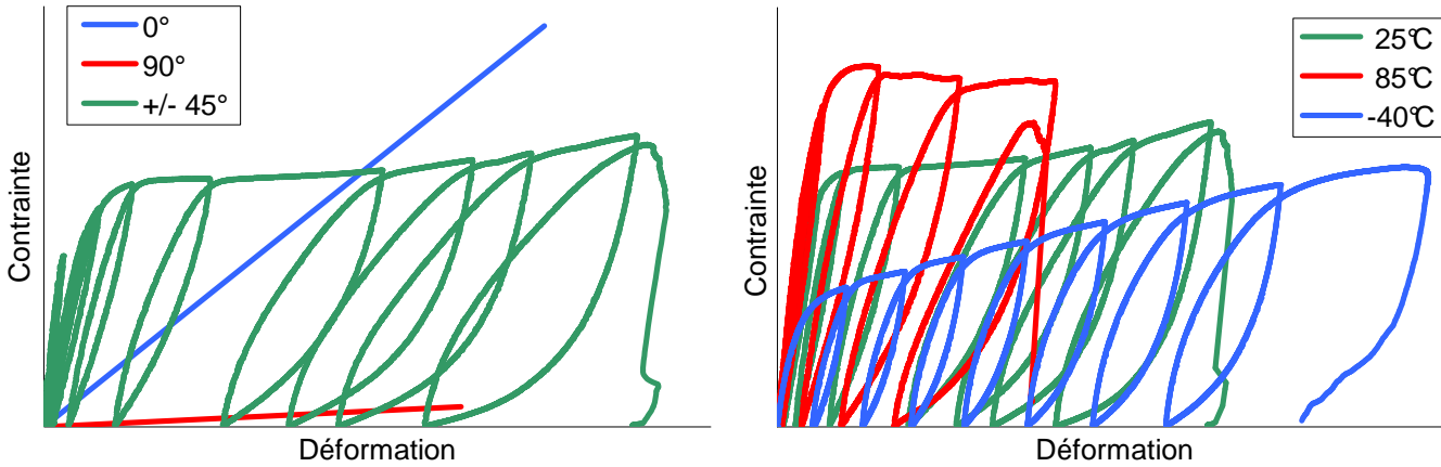
Fig. 2. Loi contrainte - déformation pour différentes orientations à 25°C (a) et Loi contrainte - déformation des +/- 45° pour différentes températures (b)
