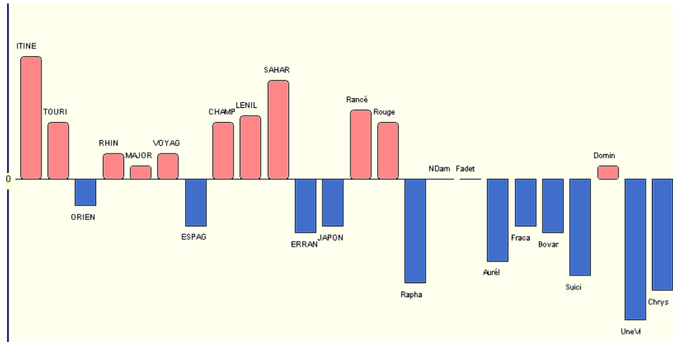
Graphique 6 – Le quotient entre le code masculin et le code féminin
