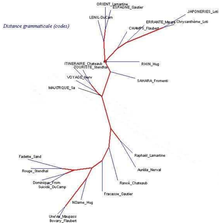
Graphique 1. La distance grammaticale (les codes)
