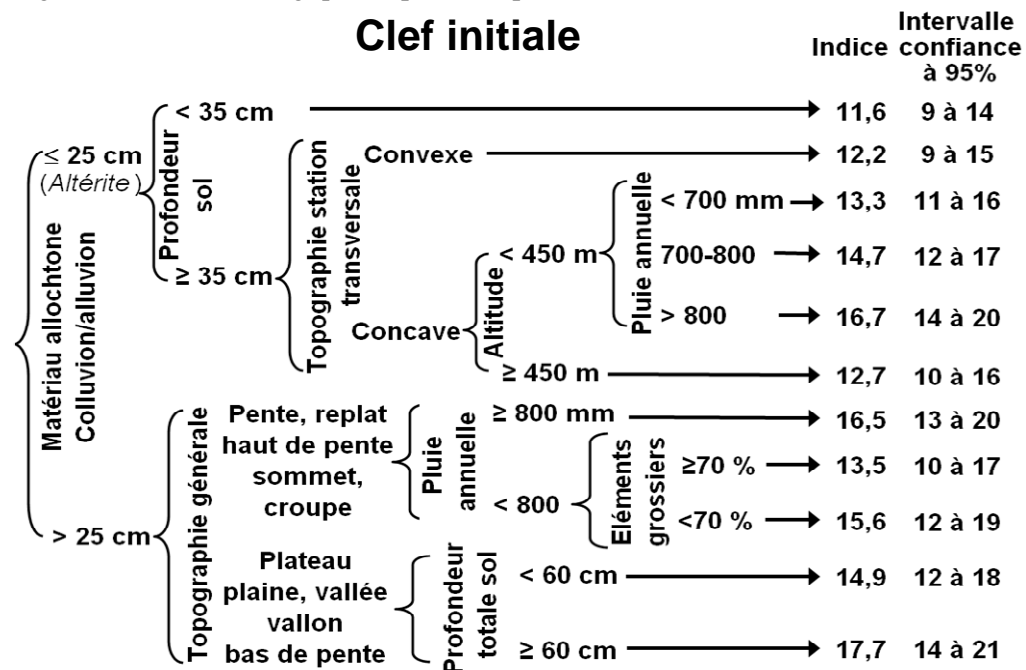
Figure 3 : Clef autécologique du pin d'Alep fondée sur le modèle en arbre de décision. La clef s'utilise en 2 à 4 étapes suivant les conditions de milieu
