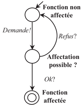
Fig. 3. Modèle générique ( \delta ) de demande d'affectation
