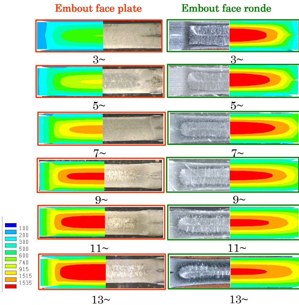
FIG. 2 - Comparaison des cinétiques de développement de noyau expérimentales et numériques dans les deux configurations électrodes neuves à embouts rayonnés et électrodes usagées à embouts aplatis.
