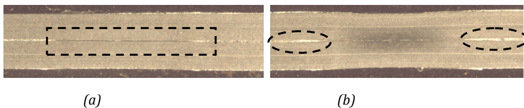
FIG. 5 - Coupes macrographiques d'un point soudé interrompu à 1~ (a) et à 2~ (b). Observation d'un espace vide entre les deux tôles (a) et d'un anneau de zinc à la périphérie du contact T/T (b).
