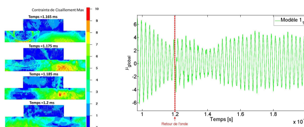
FIG. 9 – Parallèle entre la propagation des ondes dans le modèle 1_1 et l'apparition des perturbations sur l'évolution temporelle de \bar{\mu}
