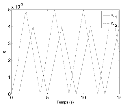
FIGURE 3 – Essai de traction-cisaillement déphasé : évolution des déformations
