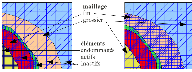
FIGURE 2 – Principe du remaillage avec zone cohésive (à gauche avant remaillage, à droite après).
