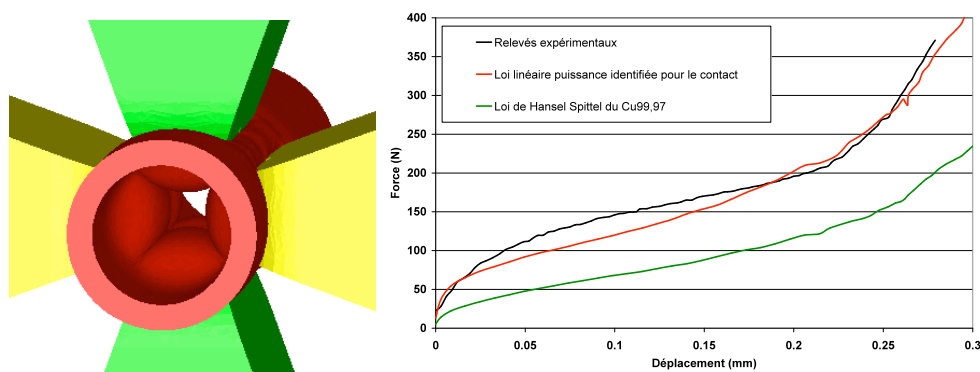
Figure 3 — Visuel du modèle d'un sertissage à vide et relevés d'efforts expérimentaux et simulés avec deux rhéologies différentes
