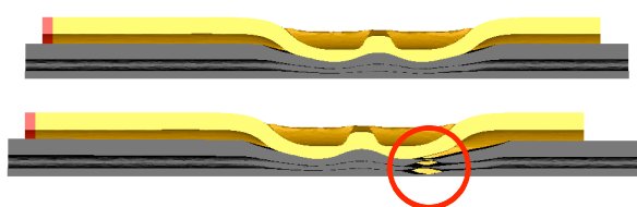
Figure 10 — Evolution de la géométrie au cours de la traction pour la configuration 2 de matériaux
