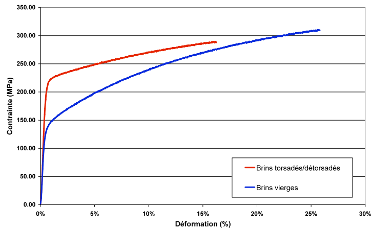
Figure 1 – Courbes contraintes/déformations obtenus par essais de traction sur brins vierges ou issus d'un câble
