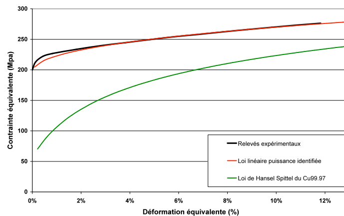
Figure 2 – Courbes contraintes/déformations obtenues expérimentalement, par simulation avec la loi linéaire puissance identifiée ou par simulation avec la loi Cu99,97
