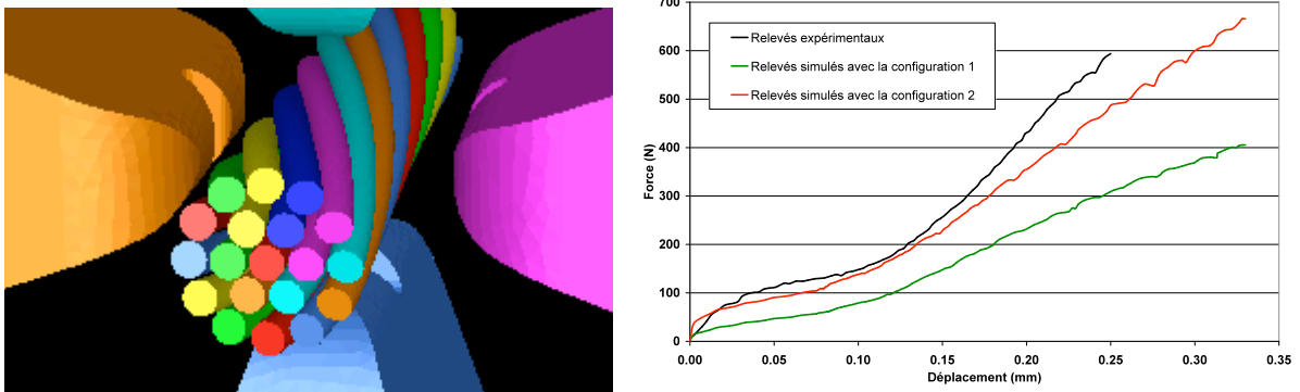
Figure 8 – Visuel du modèle complet torsadé et comparaison des efforts de sertissage expérimentaux et simulés avec deux rhéologies différentes
