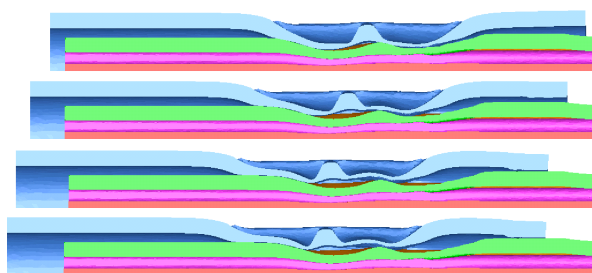
Figure 9 — Evolution de la géométrie au cours de la traction pour la configuration 1 de matériaux
