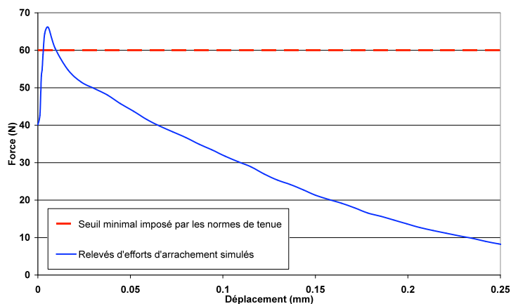
Figure 11 — Relevé d'efforts obtenu avec la configuration 2 et seuil d'admissibilité d'un contact
