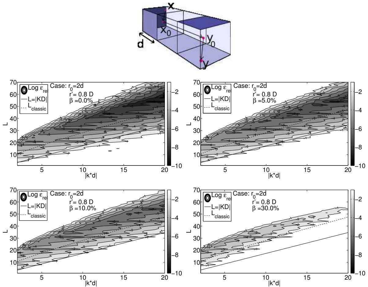
FIGURE 2 – Carte des isovaleurs de l'erreur relative \varepsilon_{rel} = |G_L - G_{an}|/|G_{an}| entre deux points fixés ( \mathbf{r}' = 0.8D ) positionnés dans deux cellules les plus proches non-adjacentes : influence de l'amortissement \beta .
