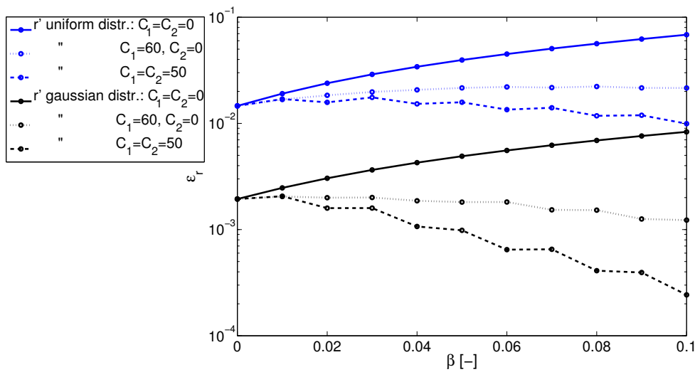
FIGURE 4 – Erreur relative dans l'approximation du noyau G pour deux distributions de nuages de points \mathbf{r}' et une distance entre cellules fixée à \mathbf{r}_0 = 2(k^*d) : influence des constantes C_1, C_2 .
