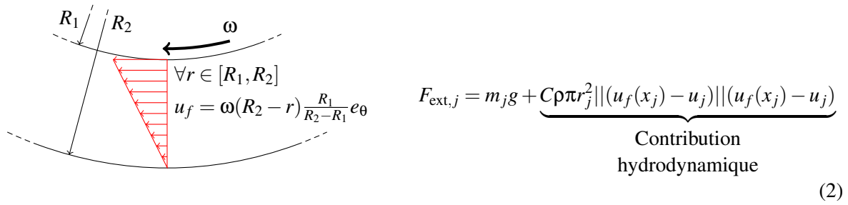
FIGURE 2 – Ecoulement de Couette cylindrique vu dans le plan (e_r, e_\theta) .
