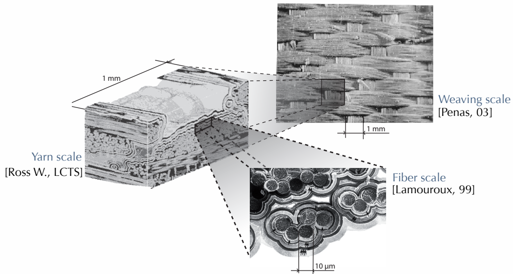
FIGURE 1 – Les différentes échelle des composites à matrice céramique.
