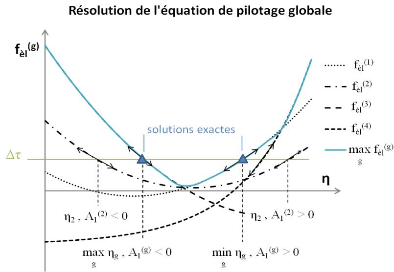
Fig. 3. algorithme de maximisation globale
