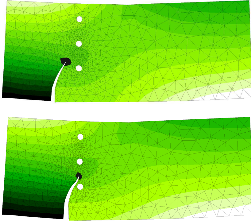
FIGURE 7 – Déformées obtenues par la méthode proposée. En noir les patch analytiques \Omega_W pour chacune des configurations au bout de 25 pas de propagation.
