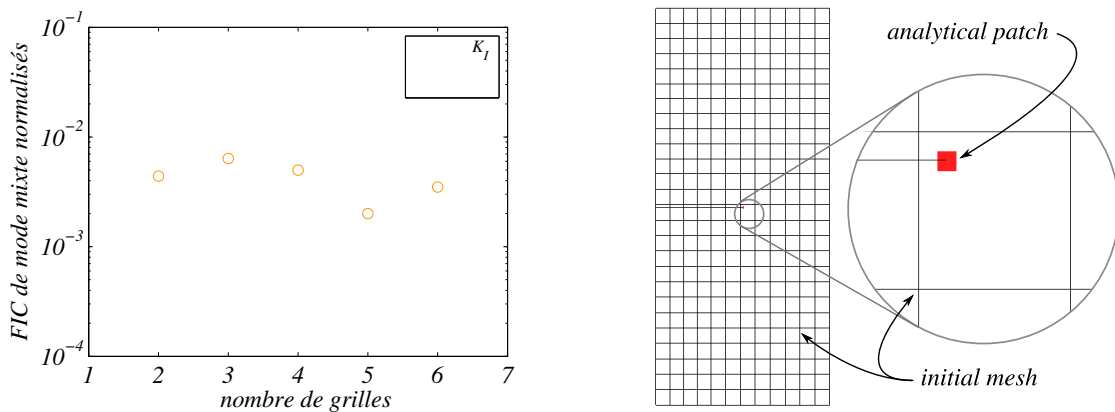
FIGURE 6 – Précision des FIC en mode mixte (à gauche) ; taille du modèle analytique et taille du maillage initial avec 4 grilles intermédiaires (à droite).
