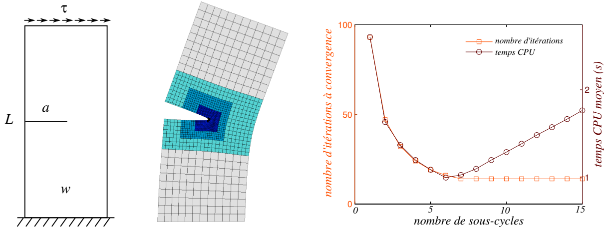
FIGURE 5 – Plaque fissurée en cisaillement : définition de la géométrie (à gauche), exemple d’une hiérarchie de 5 grilles (au centre) et solution associée en déplacement (à droite).
