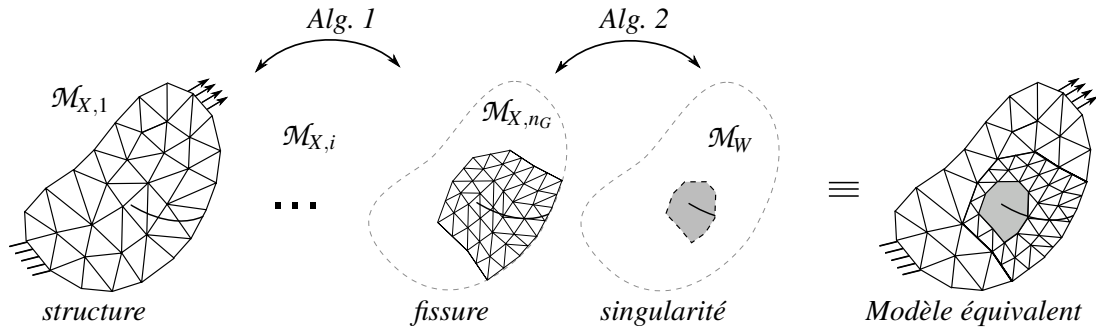
FIGURE 2 – illustration de la hiérarchie de modèles
