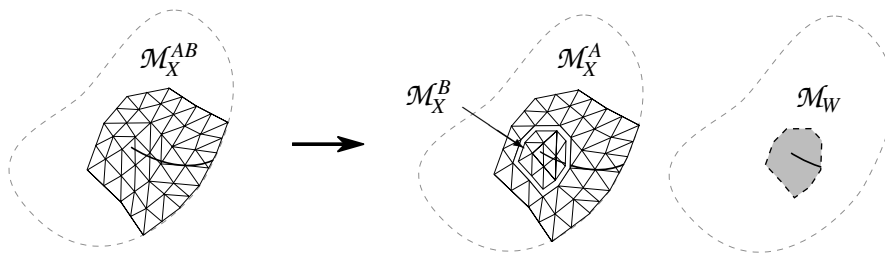
FIGURE 3 – Alg.2 : Maillage X-FEM le plus fin \overline{\mathcal{M}}_{AB} et patch analytique \mathcal{M}_W
