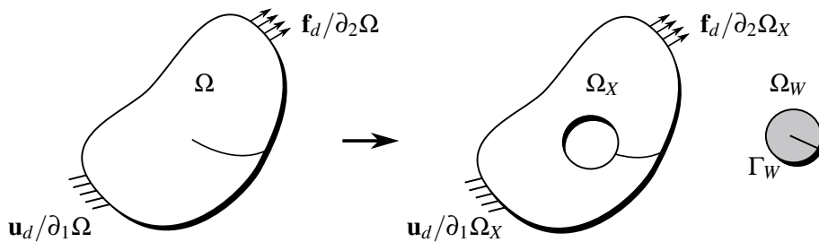
FIGURE 1 – Problème de référence et décomposition du domaine en un patch analytique et un domain X-FEM.
