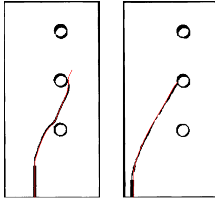
FIGURE 8 – Comparaison de la simulation avec les observations expérimentales de Bittencourt et al. [9]
