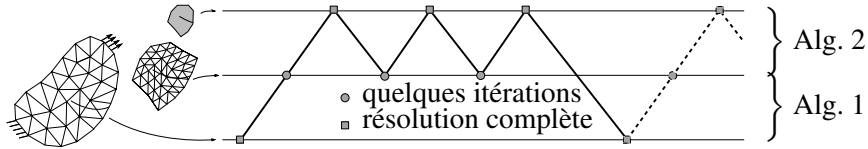
FIGURE 4 – W -Cycle multigrille élémentaire avec \gamma = 3 sous-cyclages de l'Alg. 2
