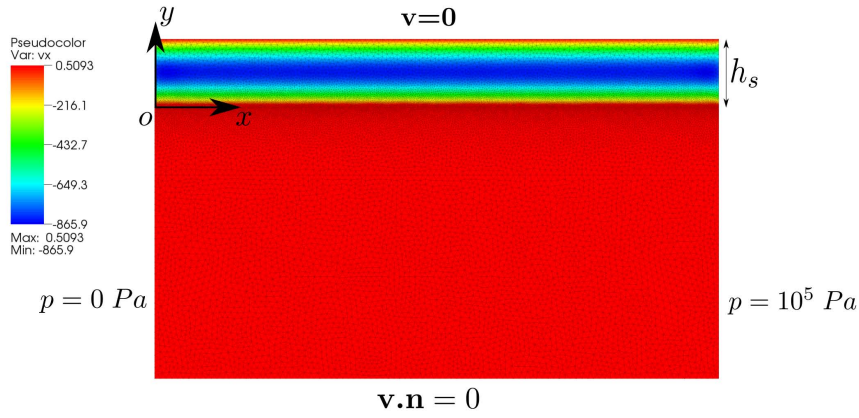
FIG. 2 – Distribution de pression et conditions aux limites pour le cas test d'écoulement tangent, avec \eta = 1 \text{ Pa.s} et K = 10^{-2} \text{ m}^2 .
