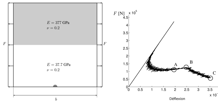
FIG. 2 – Description de la géométrie et du chargement et courbe effort déflexion
