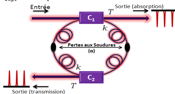
Figure 1. Résonateur optique à boucle fibrée
