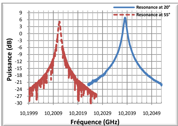
Figure 7. Décalage de 2.5 MHz de la résonance dans une boucle fibrée de 20 mètre pour \Delta T = 35 K et f_{RF} = 10.2 GHz
