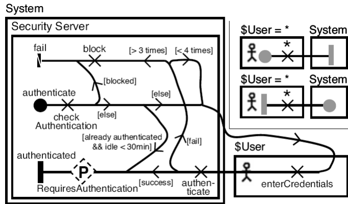
Fig. 2. AoURN model
