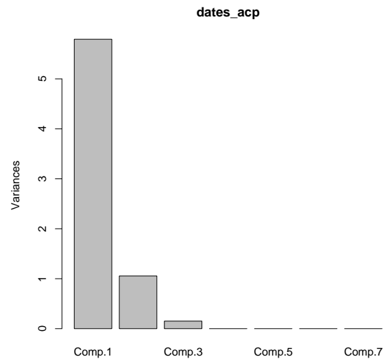
Figure 5 – Éboullis des valeurs propres de l’ACP
