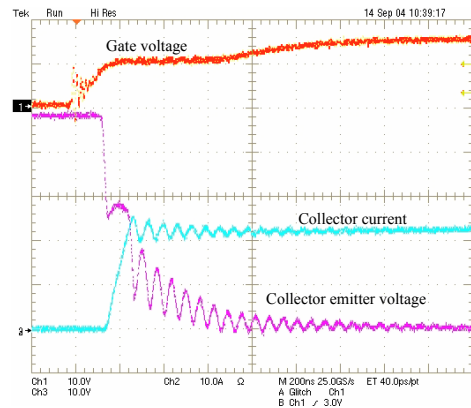
Fig. 10 - Hard-switching turn-on
