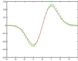
Ex 3 ( n\Delta = 1000 ) MISE= 2,7 \cdot 10^{-3} Ex 3 ( n\Delta = 10000 ) MISE= 1,4 \cdot 10^{-3}
