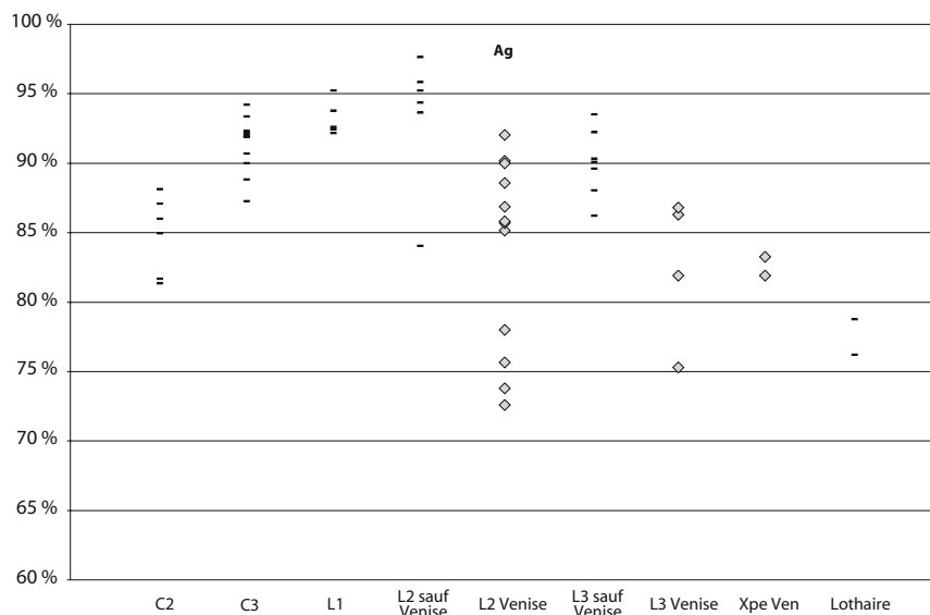
Fig. 2 - Titre des deniers d'Italie carolingienne et vénitiens analysés
