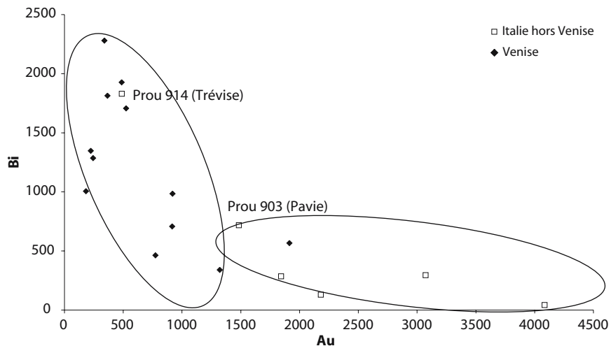
Fig. 3 - Diagramme binaire représentant les teneurs en bismuth en fonction des teneurs en or pour les deniers italiens et les deniers vénitiens. Toutes valeurs en ppm
