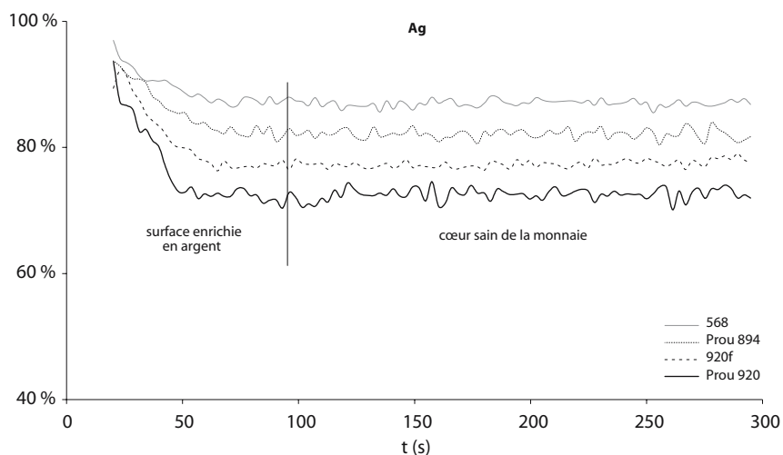
Fig. 1 - Exemples de profils de concentration obtenus sur quatre deniers carolingiens représentant l'évolution de la teneur en argent en fonction de la durée de l'ablation laser en secondes
