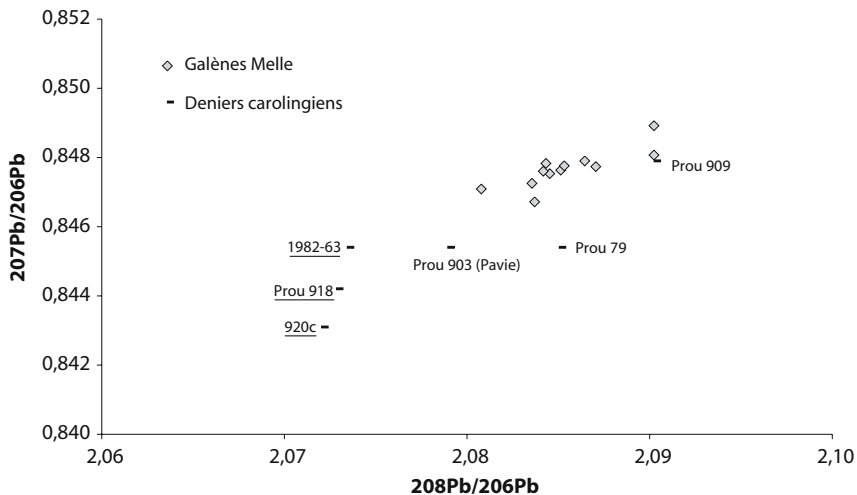
Fig. 5 – Caractéristiques isotopiques du plomb de six deniers de notre corpus. Les références soulignées correspondent aux monnaies de Venise. Les caractéristiques de galènes de la mine de Melle sont également reportées.
