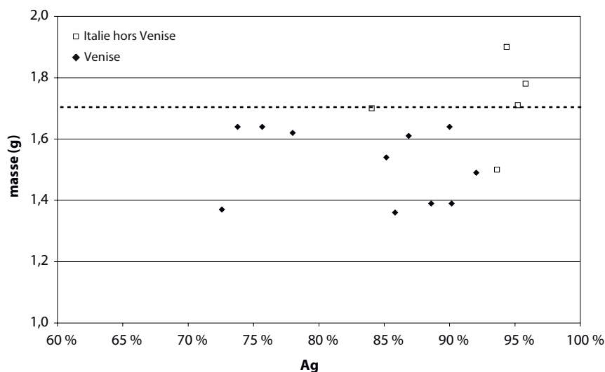
Fig. 6 - Représentation du titre des deniers carolingiens d'Italie et vénitiens frappés sous Louis le Pieux entre 818 et 822 en fonction de leur masse
