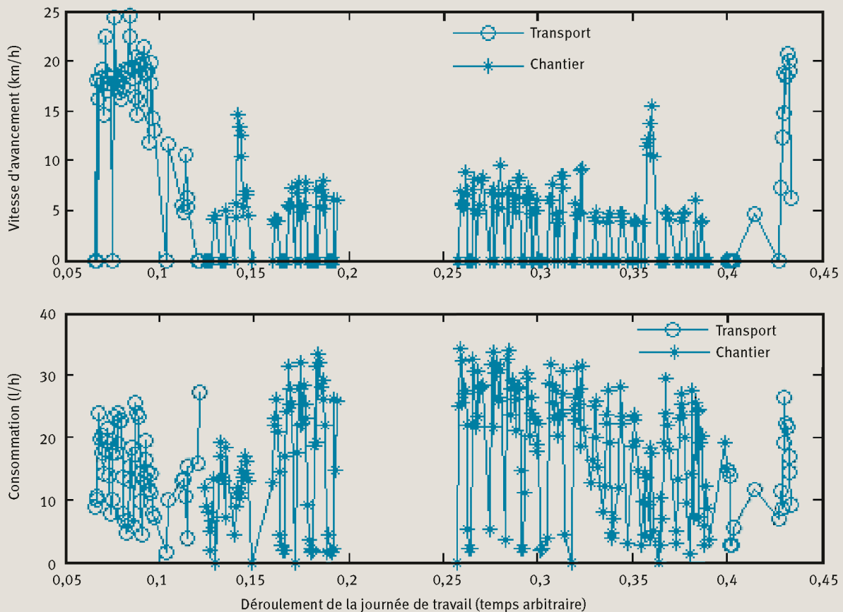
3 Vitesse d'avancement et consommation horaire mesurées au cours de la journée de travail
