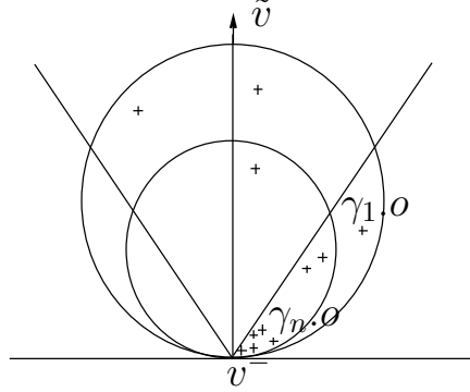
FIGURE 2 – Relevé d'un vecteur horocyclique à droite
