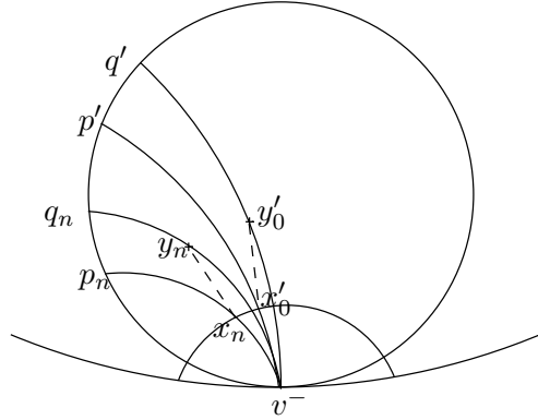
FIGURE 5 – Démonstration du théorème 1.2
