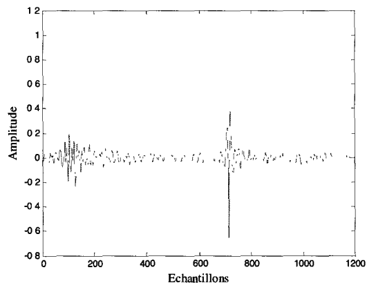
Figure IV.12: Corrélation du signal reçu avec l'impulsion de référence
