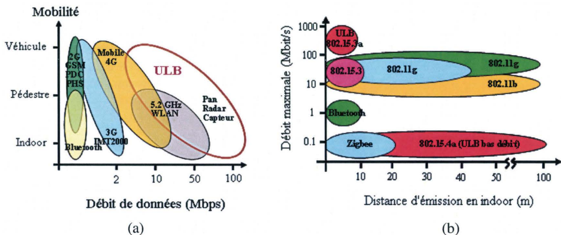
Figure II.11 : Positionnement des systèmes ULB par rapport aux systèmes existants en terme de débit et de mobilité (a), en terme de débit et de portée (b).
