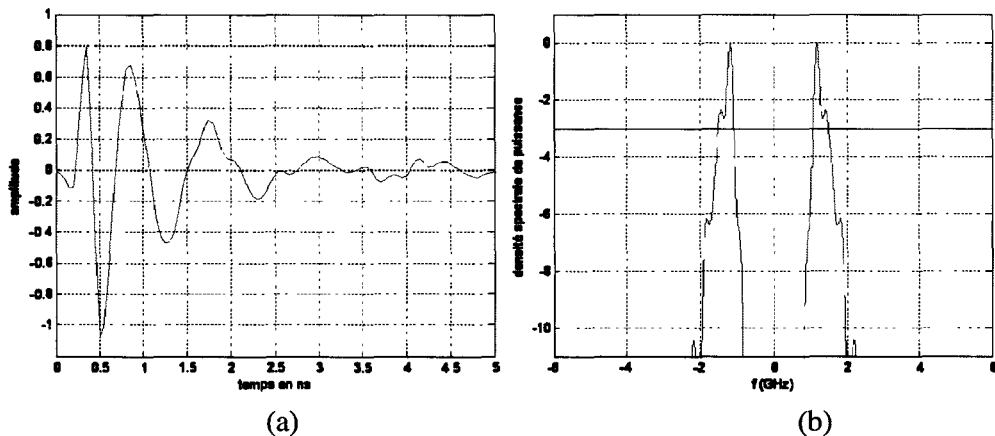
Figure V.12 : Impulsion enregistrée à vide et son spectre (20 GS/sec).
