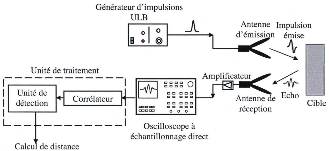
Figure IV.15 : Schéma synoptique du radar ULB réalisé
