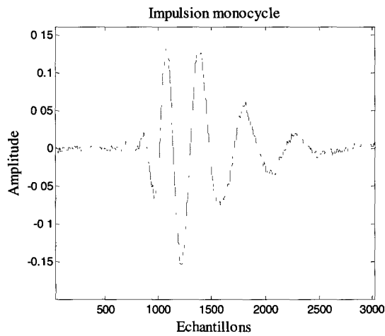
Figure IV.42: Impulsion de référence
