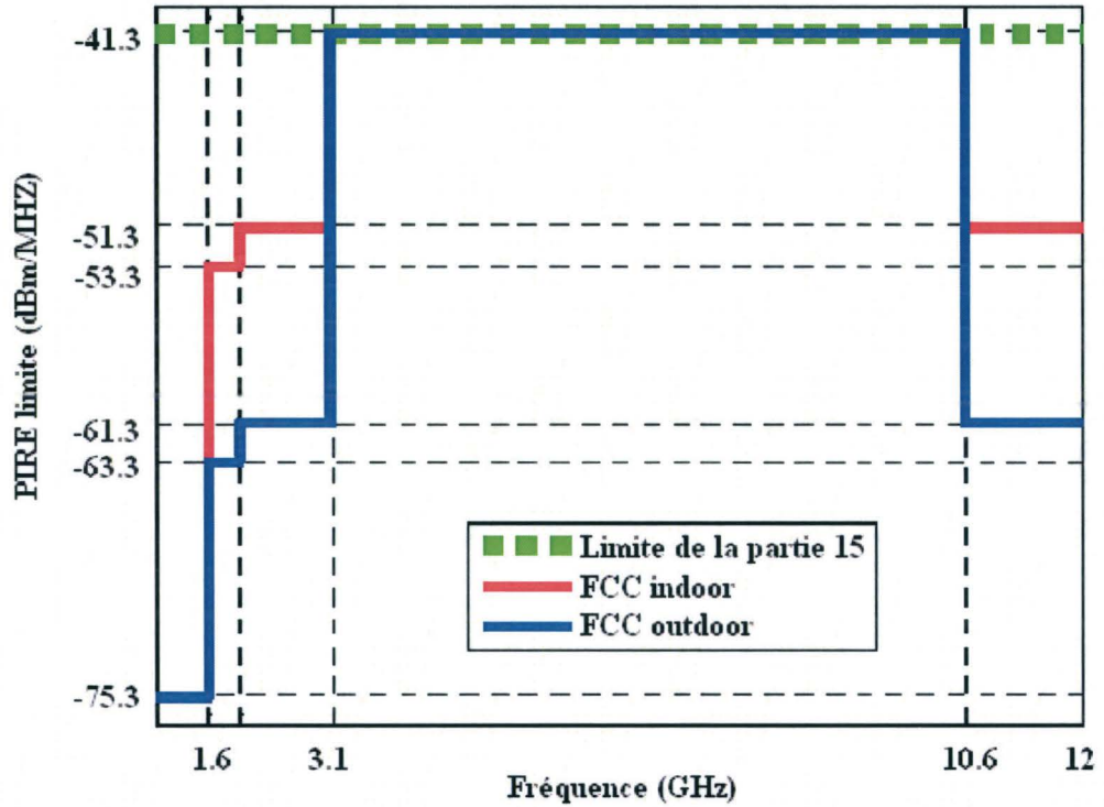
Figure II.2 : Masque d'émission des signaux ULB établi par la FCC pour les communications en intérieur (Indoor) et en extérieur (outdoor) des signaux ULB
