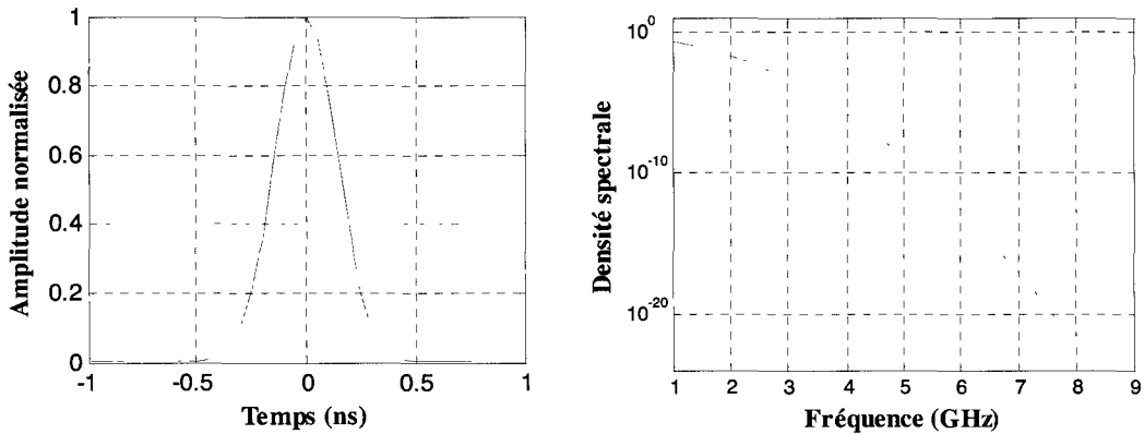
Figure III.1 : La représentation temporelle et fréquentielle de l'impulsion Gaussienne
