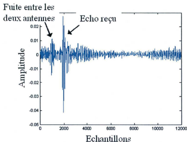
Figure IV.18 : Echo reçu de la plaque métallique placée à 1,30 m
