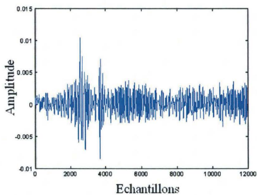
Figure IV.24 : Echo reçu de la voiture placée à 3 m
