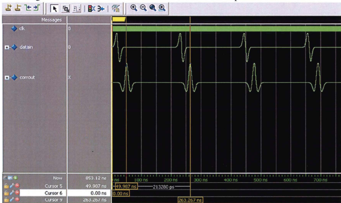
Figure V.17. Liaison du CAN avec le FPGA avec une implémentation en série.
