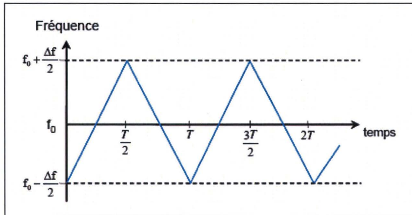
Figure I.12 : Variation de la fréquence dans le temps d'un signal LFM à modulation en toit
