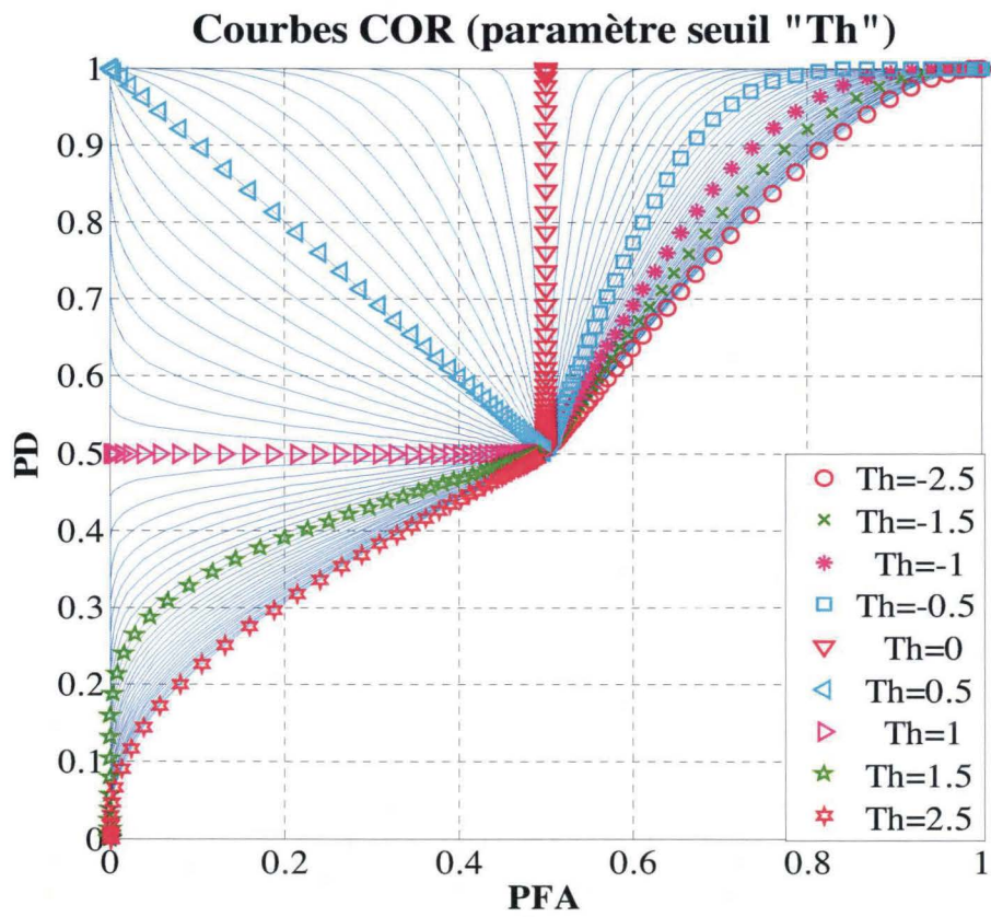
Figure IV.8: Courbes COR pour c(\tau) = 1 – Paramètre Th.
