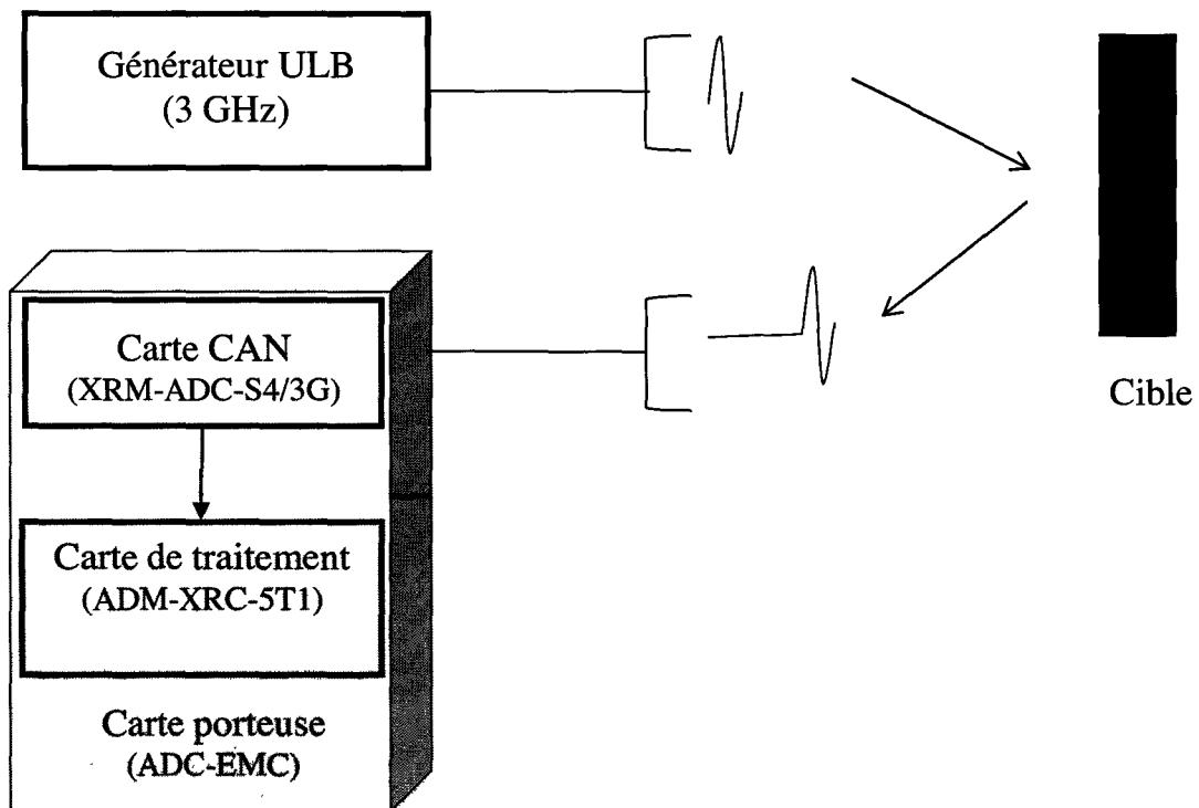
Figure V.8 : Mise en place des 3 cartes dans le système à réaliser.
