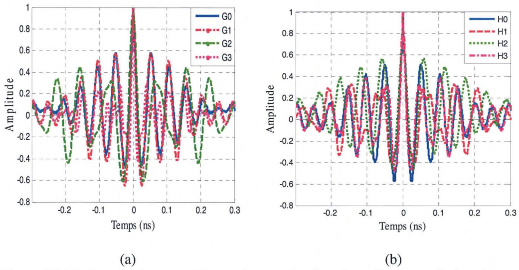
Figure III.14: Comparaison expérimentale entre les fonctions d'autocorrélation des quatre premiers ordres des fonctions de Gegenbauer (a) et d'Hermite (b)
