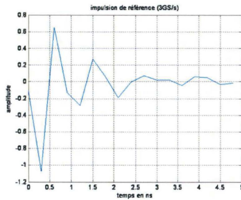
Figure V.13 : Impulsion enregistrée à vide avec une acquisition à 3 GS/sec.
