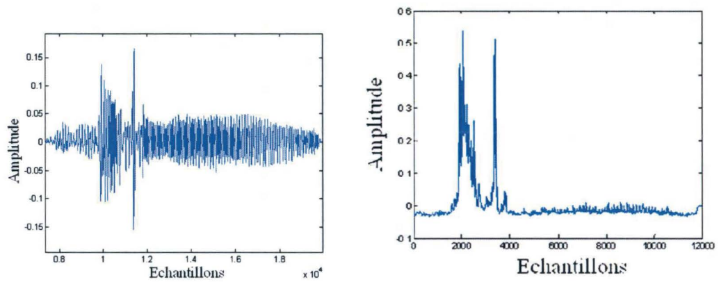
Figure IV.40 : Comparaison entre le résultat de corrélation et de l’algorithme « Tugnait » d’ordre 4 pour le piéton placé 1,70 m.
