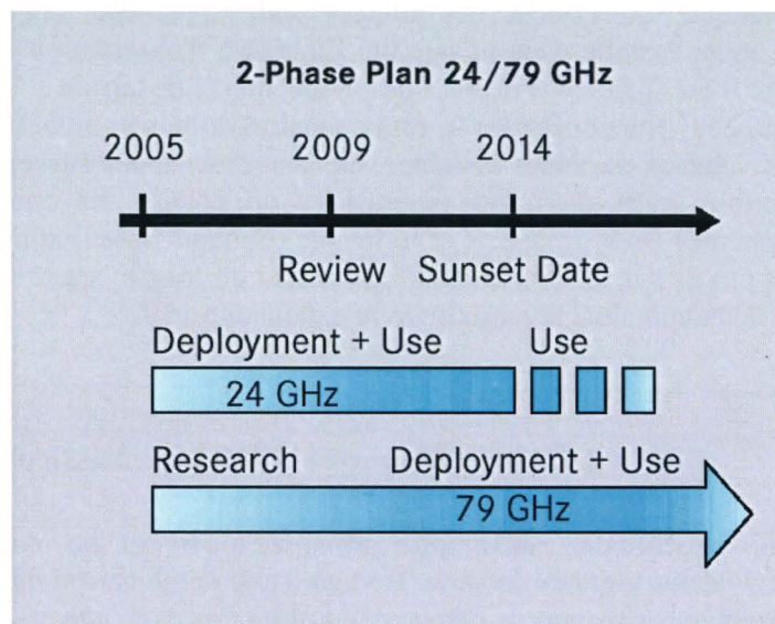
Figure II.15: Allocation de fréquences pour les radars ULB SRR en Europe
