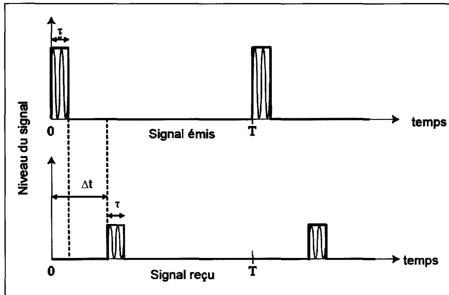
Figure I.3 : Principe du radar à impulsions
