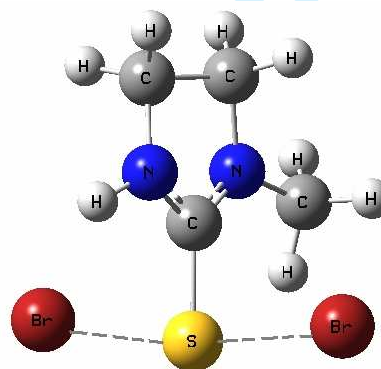
M'Br 2 T-shaped
