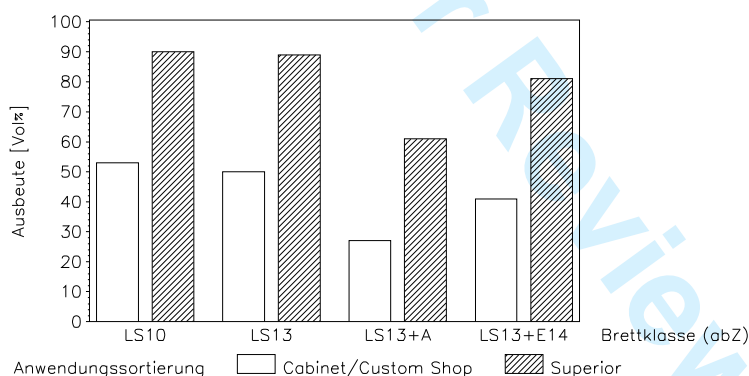
Abb. 12 Ausbeute in den Brettklassen der allgemeinen bauaufsichtlichen Zulassung (abZ)
