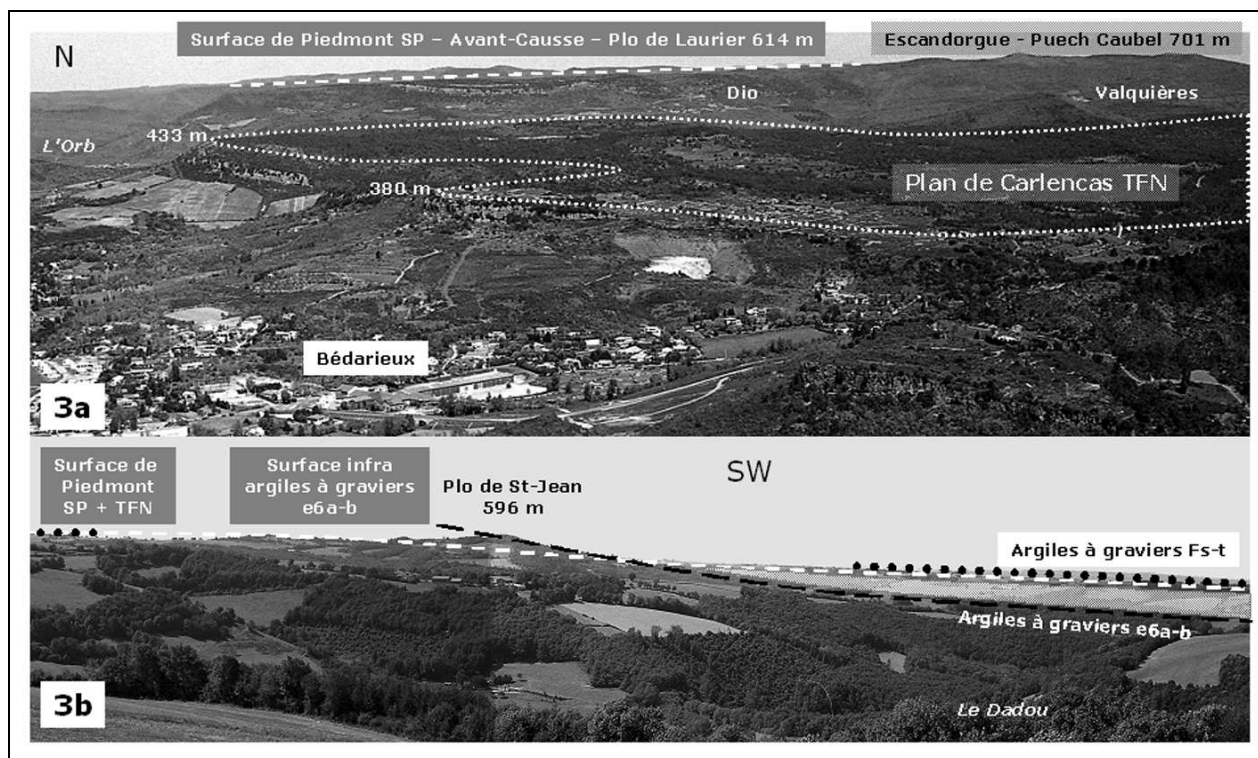
Figure 3 – L'asymétrie d'évolution morphogénétique. La topographie « fini-néogène » TFN, emboîtée de 200 m en contrebas de SP sur le piedmont languedocien (3a, depuis le Pic de Tantajo), regrade SP sur le piedmont aquitain à l'est de Réalmont (3b, depuis la D 79 en rive nord du Dadou, près de Paulinet). Clichés C. Giusti.
