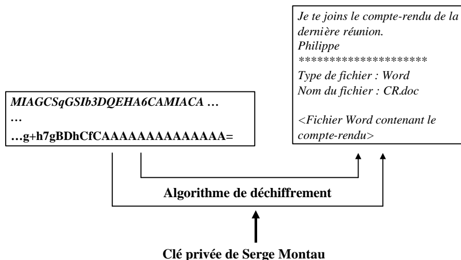
Figure 10 : déchiffrement S/MIME
