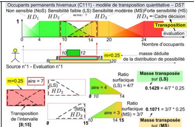
Figure 15 : Principe de la transposition par projection géométrique
