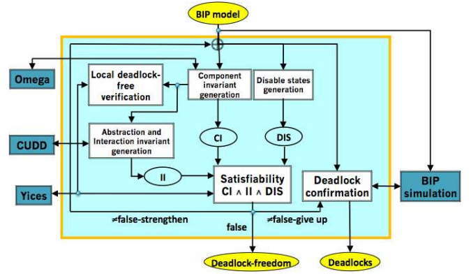
Fig. 4. D-Finder tool
