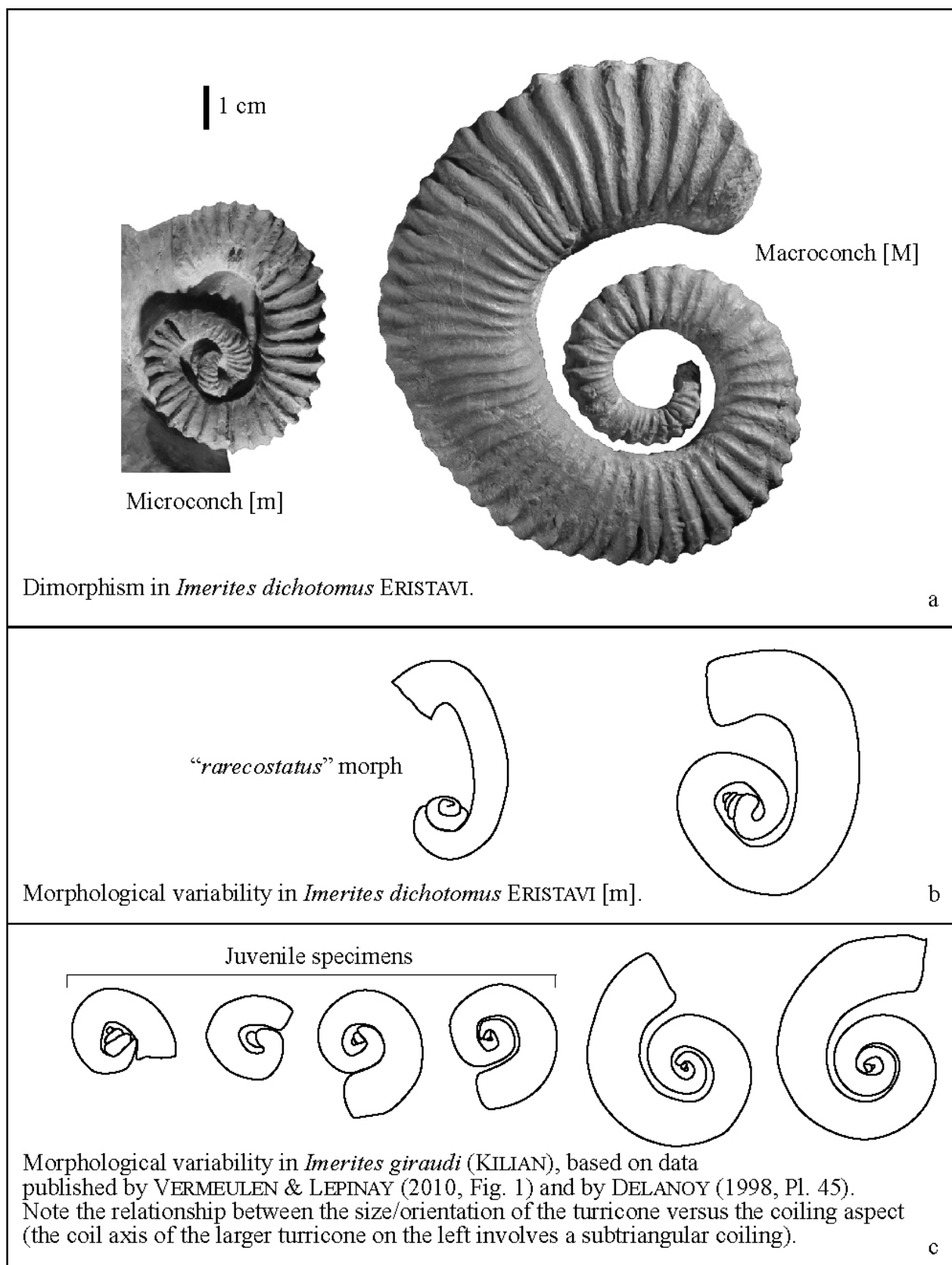
Figure 6: Dimorphism and variability in shell morphology in Imerites . Figure 6 : Dimorphisme et variabilité morphologique de la coquille chez Imerites .
