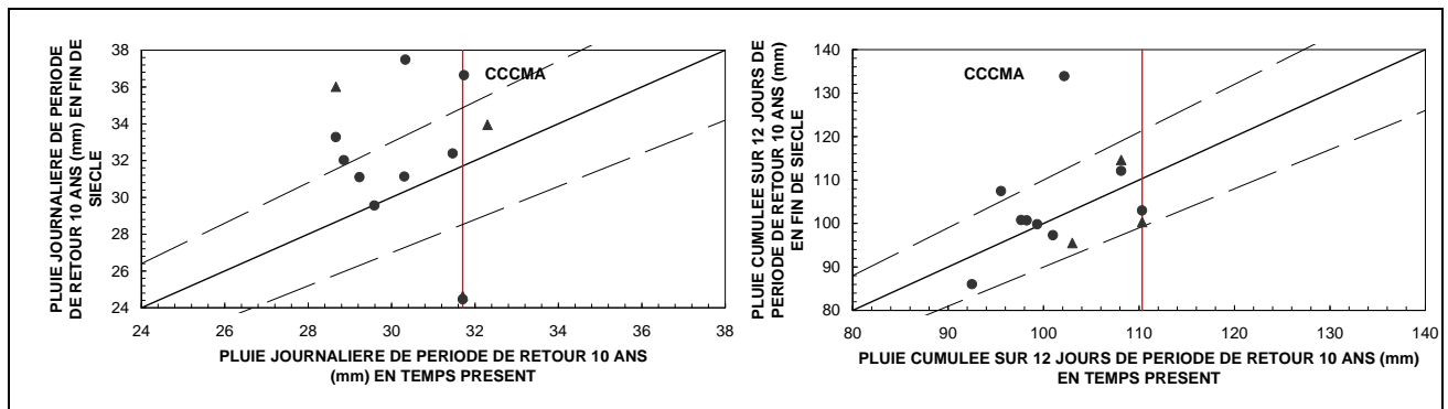
Figure 4 - Evolution des quantiles décennaux de la précipitation moyenne à l'amont de Paris entre le climat présent (PST) et la fin du siècle (FS) : maximum journalier annuel PJXA10 et maximum annuel du cumul sur 12 jours P12JXA(T=10 \text{ ans}) . Un point par scénario climatique régionalisé (● : scénarios régionalisés A1B ; ▲ : scénarios régionalisés A2 – issus du modèle climatique ARPEGE). La droite oblique est la première bissectrice et celles en tireté définissent les enveloppes à \pm 10\% des valeurs PST. La droite verticale rouge donne les quantiles décennaux déduits des précipitations SAFRAN pour la période PST.
