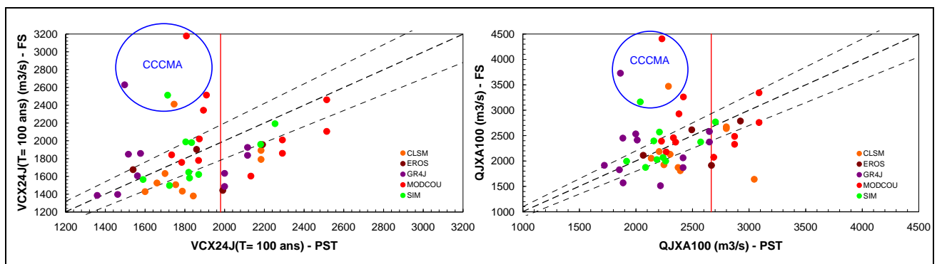
Figure 5 - Evolution des quantiles centennaux du débit à Paris entre le climat présent (PST) et la fin du siècle (FS) : débits moyens sur 24 jours VCX24J(T=100 \text{ ans}) et débits journaliers QJXA100 . Un point par scénario hydrologique. La droite en tireté est la première bissectrice et celles en pointillé définissent les enveloppes à \pm 10\% des valeurs PST. La droite verticale rouge donne les quantiles centennaux déduits des observations de débit [14].
