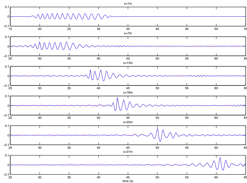
Figure 3 – 1er cas : (1.3Hz à 0.8Hz) : Comparaison entre les résultats du modèle (ligne bleue continue) et l'expérience (pointillé rouge) pour la surface libre à différents fetchs (en m) avec vent ( U=6\text{m/s} ).
