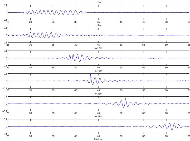
Figure 2 – 1er cas : (1.3Hz à 0.8Hz) : Comparaison entre les résultats du modèle (ligne bleue continue) et l'expérience (pointillé rouge) pour la surface libre à différents fetchs (en m) sans vent ( U=0\text{m/s} ).
