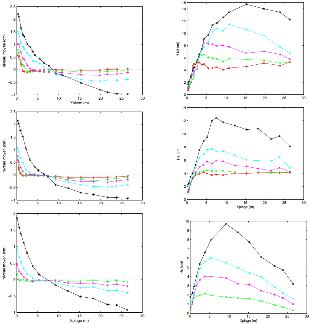
Figure 5 – (en haut) Houle régulière + vent, (au milieu) houle irrégulière + vent, (en bas) vent seul. Niveau moyen (à gauche), Hauteur significative (à droite). En rouge : houle seule, en vert : + 5m/s, en rose : + 8m/s, en bleu : + 11m/s, en noir : + 15m/s).
