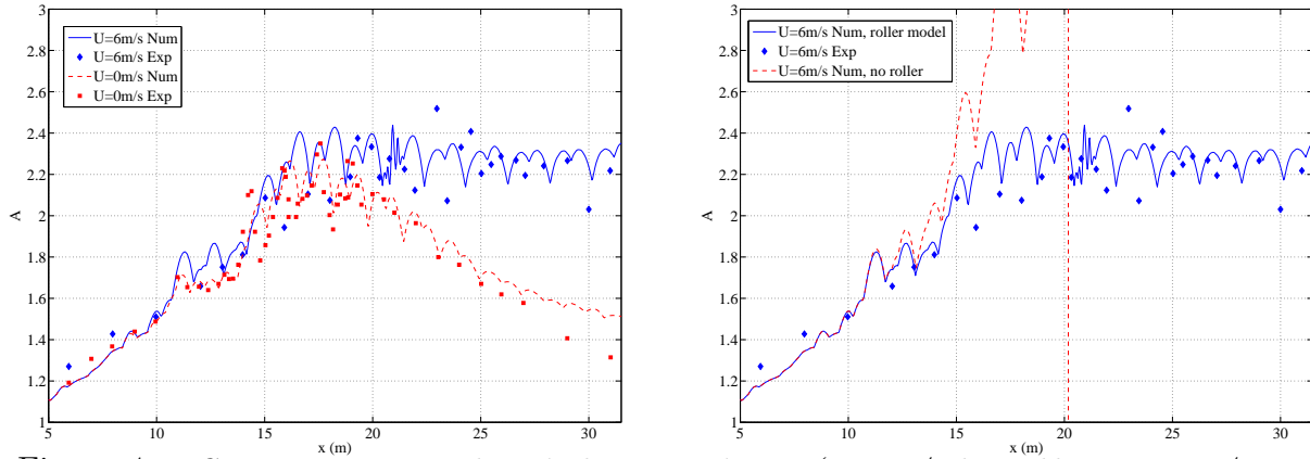
Figure 4 – Comparaison entre les résultats numérique ( U=0\text{m/s} ligne bleue, U=6\text{m/s} pointillé rouge) et les résultats expérimentaux ( U=0\text{m/s} carré rouge, U=6\text{m/s} losange bleu) pour l'évolution du facteur d'amplification A(x,t) en fonction du fetchs (en m). Influence de la dissipation dû au déferlement (à droite).
