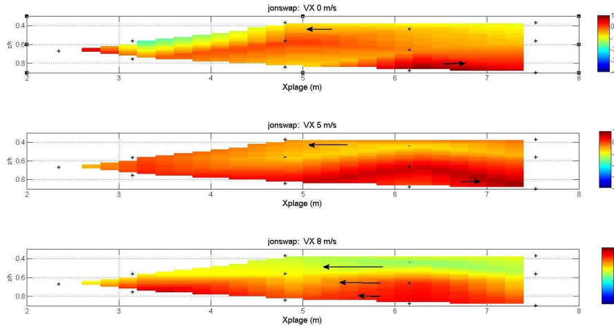
Figure 6 – profils de vitesse (cm/s) à l'abord du rivage pour une houle irrégulière.
