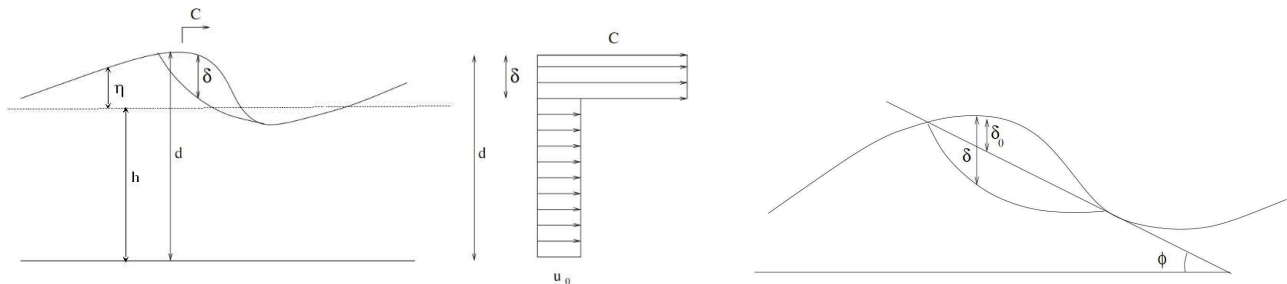
Figure 1 – Sch  ma de d  finition du roller (   gauche) et profil vertical de la vitesse associ  e (au milieu). D  tail de la m  thode (   droite).
