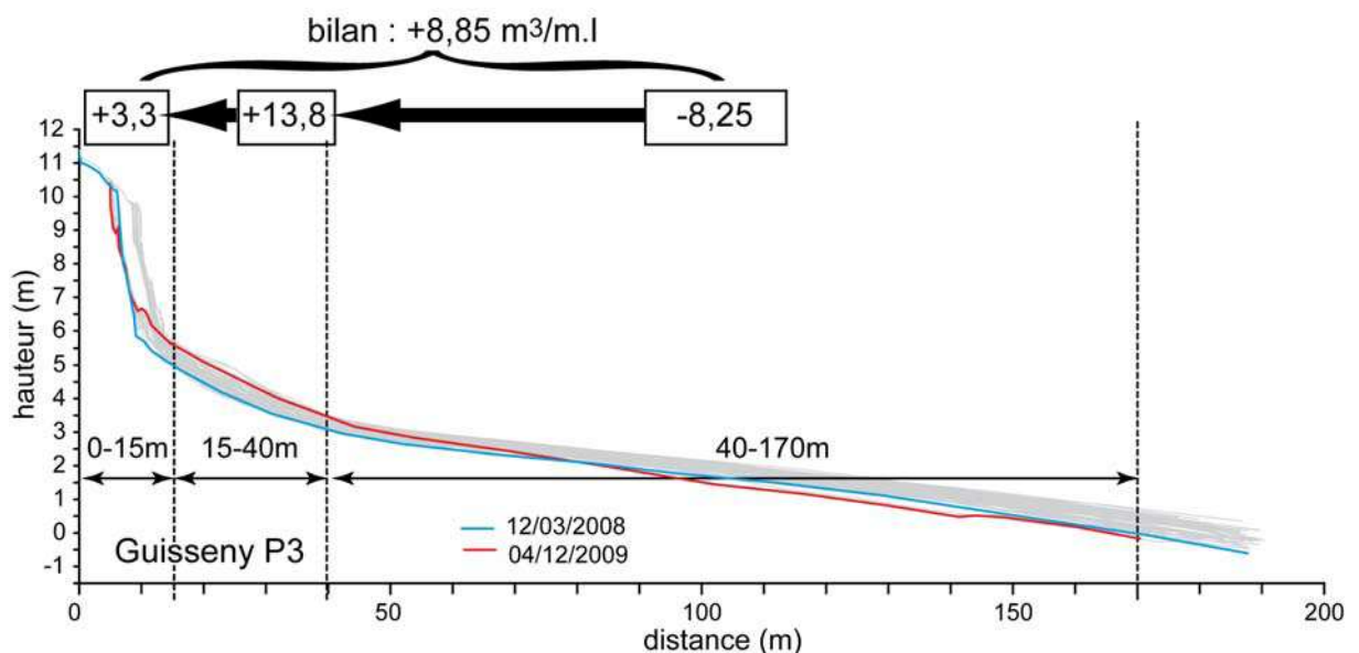
Figure 7 – Transferts sédimentaires le long de la radiale 3 et bilan sédimentaire des trois sections du profil : dune, haut de plage et bas de plage intertidale depuis la tempête du 10 mars 2008
