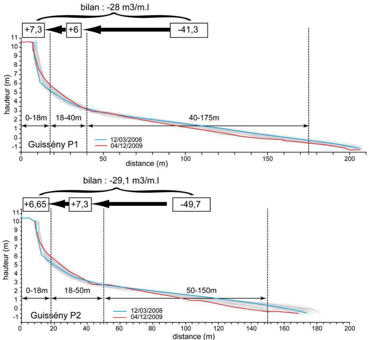
Figure 6 – Transferts sédimentaires le long des radiales 1 et 2 et bilan sédimentaire des trois sections du profil : dune, haut de plage et bas de plage intertidale depuis la tempête du 10 mars 2008
