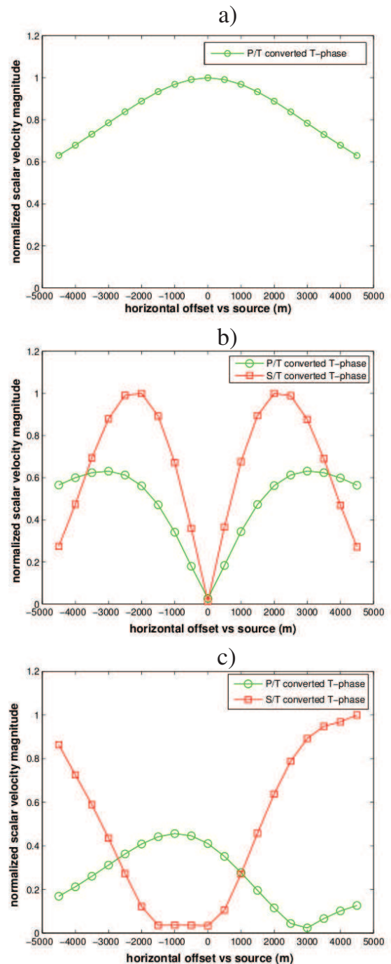
Figure 3 : maxima normalisés du module de la vitesse le long de la ligne « récepteurs » située à 500m au dessus de l'interface. a) Source explosive, b) Source double-couple 0^\circ c) Source double-couple 30^\circ . Figure reprise de [17]
