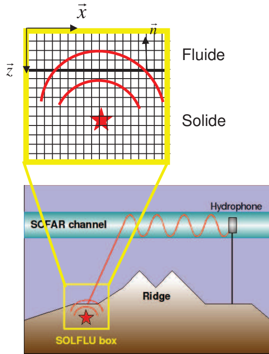
Figure 1 : Schéma de principe de la modélisation de la conversion sismique/hydroacoustique par le code en éléments finis SOLFLU. L'interface solide-fluide est orientée par le vecteur unitaire \vec{n} . Figure reprise et adaptée [17]
