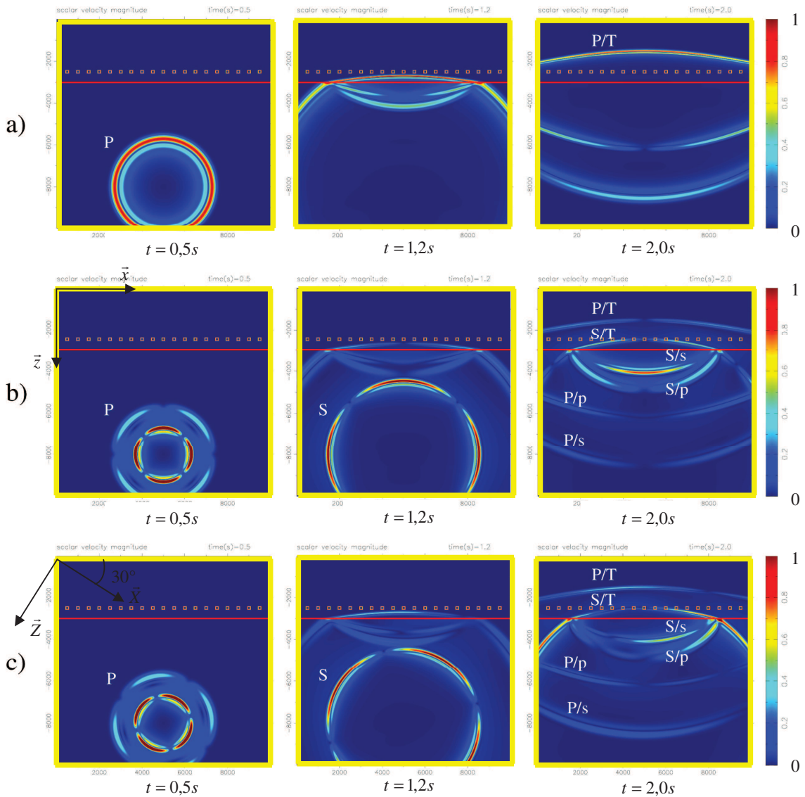
Figure 2 : Champ du module de vitesse normalisé aux instants 0.5s, 1.2s et 2.0s a) Source explosive, b) Source double-couple 0^\circ c) Source double-couple 30^\circ . La ligne rouge horizontale représente l'interface solide-fluide. Les points « récepteurs » placés à 500m au dessus de l'interface sont matérialisés par les petits carrés. Les dimensions du domaine de calcul, la position de la source, ainsi que les paramètres définissant le solide et le fluide sont donnés dans la table 1. Les ondes P et S sont les ondes directes. Les ondes P/p , P/s , S/p et S/s sont les ondes réfléchies. Les ondes P/T et les ondes S/T sont les ondes converties, respectivement les ondes P transmises et les ondes S transmises. Figure reprise [17]
