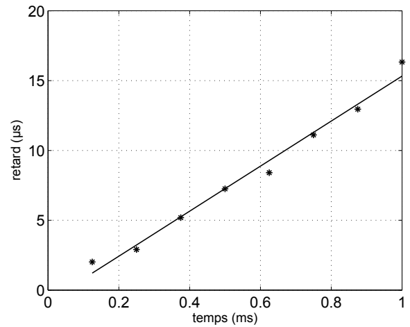
FIG. 5 – Loi de retard estimée à partir de l'intercorrélation entre deux signaux à T = 20^\circ\text{C} et T = 30^\circ\text{C} (*) et les moindres carrés correspondants (—).
