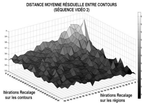
Fig. 5: Erreur moyenne résiduelle de la distance entre contours (l'axe vertical) par rapport au nombre d'itérations de recalage sur les régions et de recalage sur les contours (axes horizontaux) obtenue sur la séquence vidéo 2. Les expérimentations sur les séquences vidéo 1, 3, 4, 5 et 6 donnent des résultats similaires.
